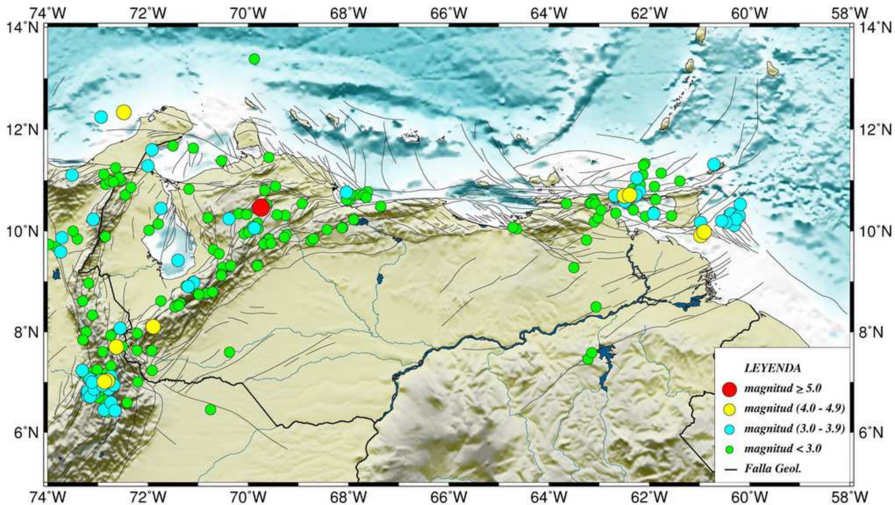
Figura 1. Mapa de ubicación geográfica de epicentros localizados durante noviembre de 2009, representado por círculos de acuerdo con el rango de magnitud asociada a cada evento. También se muestran las fallas geológicas de la región.
