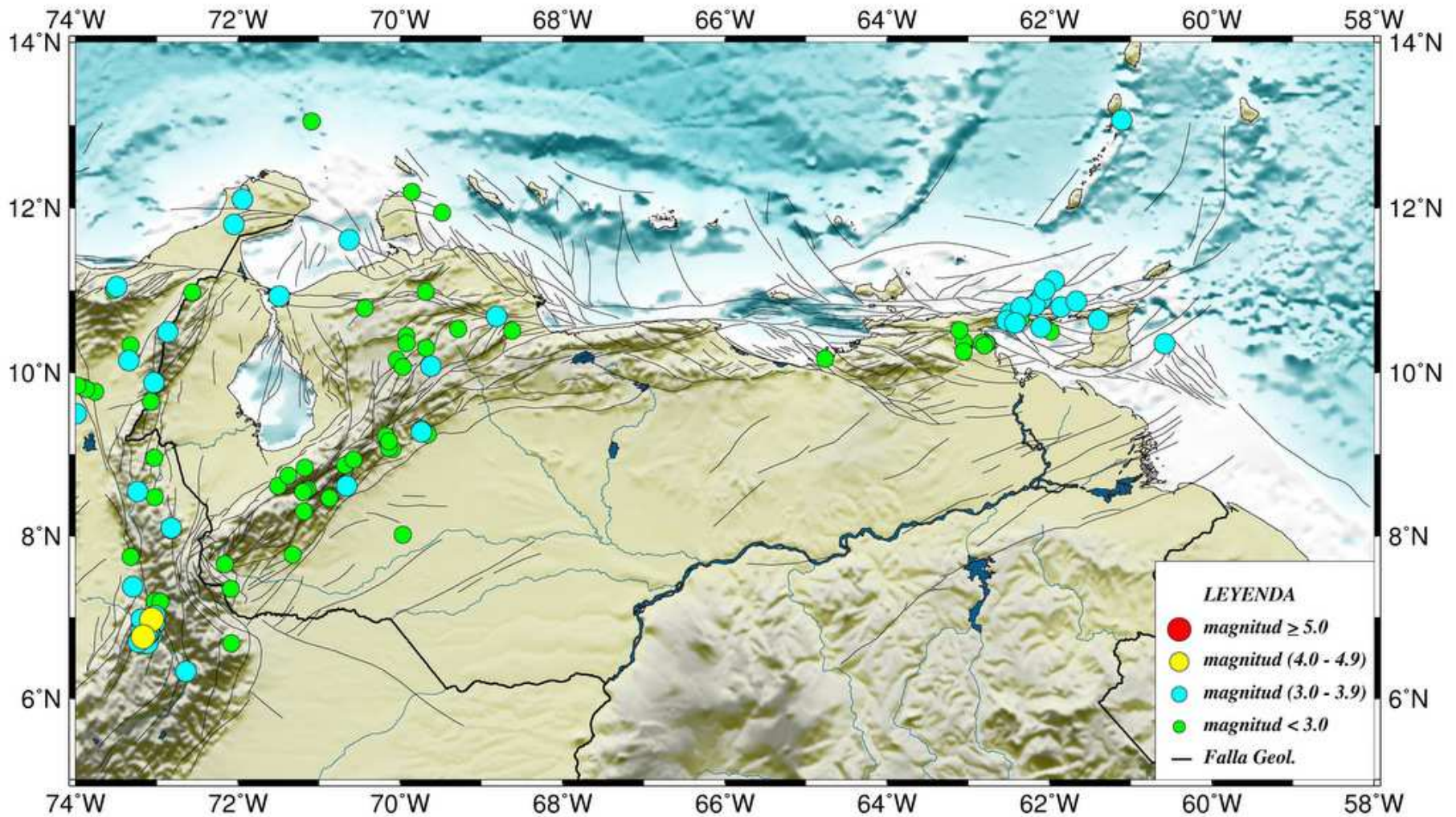
Figura 1. Mapa de ubicación geográfica de epicentros localizados durante febrero de 2009, representado por círculos de acuerdo con el rango de magnitud asociada a cada evento. También se muestran las fallas geológicas de la región.
